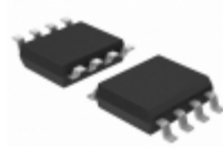
BM520Q15F-GE2 Rohm Semiconductor IC CTRL AC/DC 650V FET SOP8
