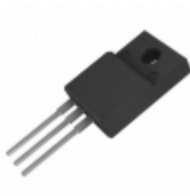
DURF1040CT Littelfuse Inc. DIODE RECTIFIER 5A 400V ITO220AB
