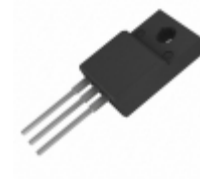
DURF1030CTR Littelfuse Inc. DIODE RECTIFIER 5A 300V ITO220AB
