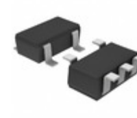
BD5328G-TR Rohm Semiconductor IC DETECTOR VOLT 2.8V CMOS 5SSOP
