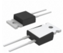
PF2203-1K8F1 Riedon RES 1.8K OHM 35W 1% TO220
