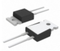
PF2203-1K3F1 Riedon RES 1.3K OHM 35W 1% TO220
