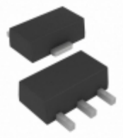
MCP112T-315E/MB Microchip Technology IC VOLT DET 3.08V LOW SOT89-3
