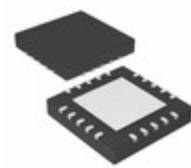
PIC18F14K50-I/MQ Microchip Technology IC MCU 8BIT 16KB FLASH 20QFN
