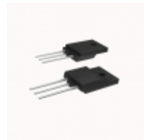
FMN-4306S SanKen Electric Co., Ltd. DIODE ARRAY GP 600V 15A TO3PF
