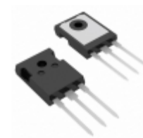
IXGH20N60AU1 IXYS IGBT 600V 40A 150W TO247AD
