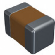
CDR31BX471BKMSAJ Electro-Films (EFI) / Vishay CAP CER 470PF 100V BX 0805
