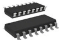
4816P-2-132LF Bourns Inc. RES ARRAY 15 RES 1.3K OHM 16SOIC
