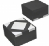
RT9080-33GQZ Richtek USA Inc. IC REG LDO 3.3V 0.6A 4ZQFN
