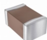
08051C102KAJ2A AVX Corporation CAP CER 1000PF 100V X7R 0805
