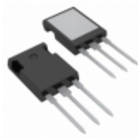
IXFR102N30P IXYS MOSFET N-CH 300V 60A ISOPLUS247
