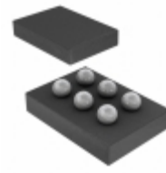
DC6M503X6/12A,135 NXP USA Inc. IC REG BCK 1.2V 0.5A SYNC 6WLCSP
