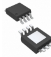
RT9069-90GSP Richtek USA Inc. IC REG LDO 9V 0.2A 8SOP
