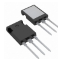
IXFR44N50Q IXYS MOSFET N-CH 500V 34A ISOPLUS247
