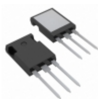
IXFR34N80 IXYS MOSFET N-CH 800V 28A ISOPLUS247
