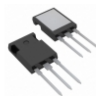
IXFR44N50P IXYS MOSFET N-CH 500V 24A ISOPLUS247
