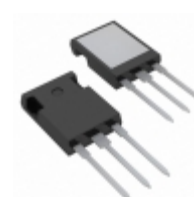
IXFR44N60 IXYS MOSFET N-CH 600V 38A ISOPLUS247
