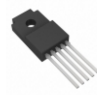
BAJ0CC0WT-F Rohm Semiconductor IC REG LDO 10V 1A TO220FP-5
