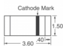
DL5254B-TP Micro Commercial Co DIODE ZENER 27V 500MW MINIMELF
