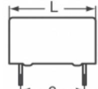
B32676G3256K000 EPCOS CAP FILM 25UF 10% 300VDC RADIAL
