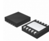
RT9018A-25GQW Richtek IC REG LDO 2.5V/ADJ 3A 10WDFN
