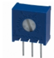
3386C-1-504 Bourns, Inc. TRIMMER 500KOHM 0.5W PC PIN SIDE
