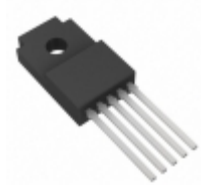
BA15BC0WT LAPIS Semiconductor IC REG LDO 1.5V 1A TO220FP-5
