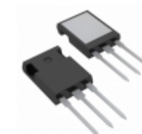
IXFR180N06 IXYS MOSFET N-CH 60V 180A ISOPLUS247
