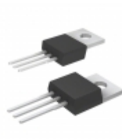
DSSK48-003B IXYS DIODE ARRAY SCHOTTKY 30V TO220AB
