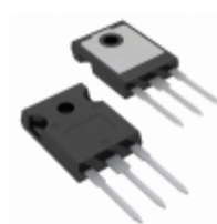
IRGP6660D-EPBF Infineon Technologies IGBT 600V 60A TO247AD
