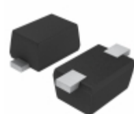
EDZTE614.7B LAPIS Semiconductor DIODE ZENER 4.7V 150MW EMD2
