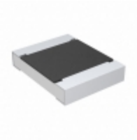
CRCW1210226KFKEA Vishay Dale RES SMD 226K OHM 1% 1/2W 1210
