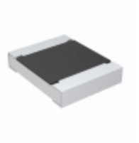
CRCW1210221RFKTC Vishay Dale RES SMD 221 OHM 1% 1/2W 1210
