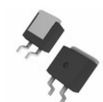
DGS20-018AS IXYS DIODE SCHOTTKY 180V 23A TO263AB
