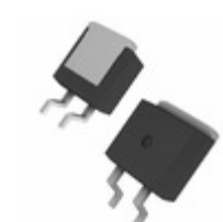
DGS20-018AS-TUBE IXYS DIODE SCHOTTKY 180V 23A TO263AB
