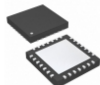
PIC24FV16KA302-E/ML Microchip Technology IC MCU 16BIT 16KB FLASH 28QFN
