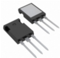
IXFR15N100Q3 IXYS MOSFET N-CH 1000V 10A ISOPLUS247
