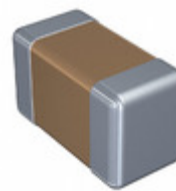
C0603C151J3HAC7867 KEMET CAP CER 0603 150PF 25V ULTRA STA
