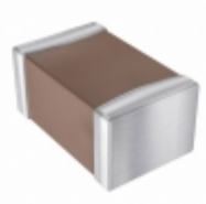
08053C224JAT2A AVX Corporation CAP CER 0.22UF 25V X7R 0805
