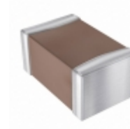
08053C224KA12A AVX Corporation CAP CER 0.22UF 25V X7R 0805
