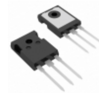
IXKH70N60C5 IXYS MOSFET N-CH 600V 70A TO247AD
