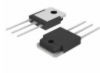
DPG60C200QB IXYS DIODE ARRAY GP 200V 30A TO3P
