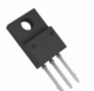
BA17809CP-E2 Rohm Semiconductor IC REG LDO 9V 1A TO220CP-3
