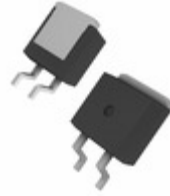
DPG60C300PC IXYS DIODE ARRAY GP 300V 30A TO263
