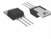
L4008L8TP Littelfuse Inc. TRIAC SENS GATE 400V 8A TO220
