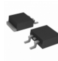
Q8010N4TP Littelfuse Inc. TRIAC 800V 10A TO263
