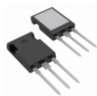
IXFR48N50Q IXYS MOSFET N-CH 500V 40A ISOPLUS247
