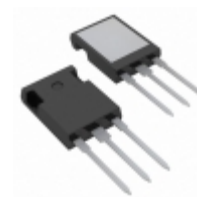
IXFR64N50Q3 IXYS MOSFET N-CH 500V 45A ISOPLUS247
