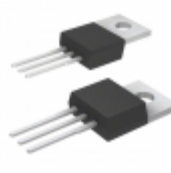
IXKP13N60C5 IXYS MOSFET N-CH 600V 13A TO220AB
