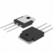
IXFQ14N80P IXYS MOSFET N-CH 800V 14A TO-3P
