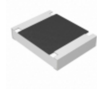
ERJ-14YJ102U Panasonic RES SMD 1K OHM 5% 1/2W 1210
