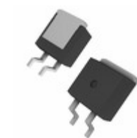
DSS16-0045AS-TUB IXYS DIODE SCHOTTKY 45V 16A TO263AB
