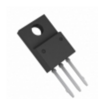
BA7809CP-E2 LAPIS Semiconductor IC REG LDO 9V 1A TO220CP-3
