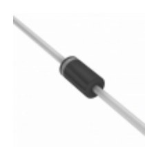
1N4745A-TR Electro-Films (EFI) / Vishay DIODE ZENER 16V 1.3W DO41
