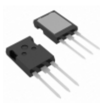
IXFX24N90Q IXYS MOSFET N-CH 900V 24A PLUS 247
