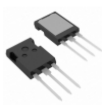
IXFX250N10P IXYS MOSFET N-CH 100V 250A PLUS247
