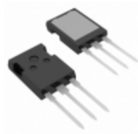
IXFX50N50 IXYS MOSFET N-CH 500V 50A PLUS247
