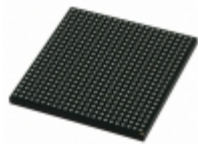
MCIMX515CJM6CR2 NXP USA Inc. IC MPU I.MX51 600MHZ 529BGA
