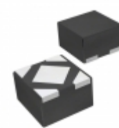
BU28JA2MNVX-CTL Rohm Semiconductor IC REG LDO 2.8V 0.2A 4SSON
