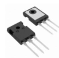
IXKH70N60C5 IXYS MOSFET N-CH 600V 70A TO247AD
